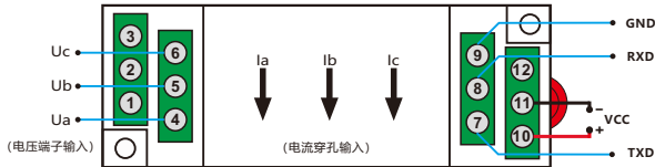
RS-232接线图：
