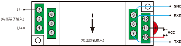
RS-232接线图：
