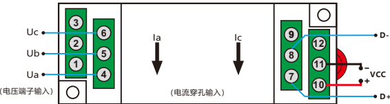
RS-485接线图：
