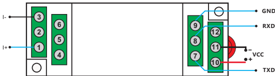
RS-232接线图：
