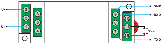
RS-232接线图：
