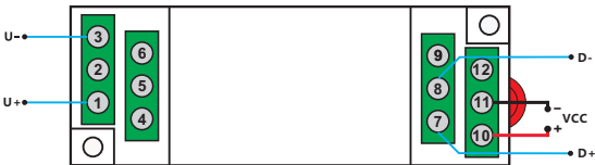
RS-485接线图：
