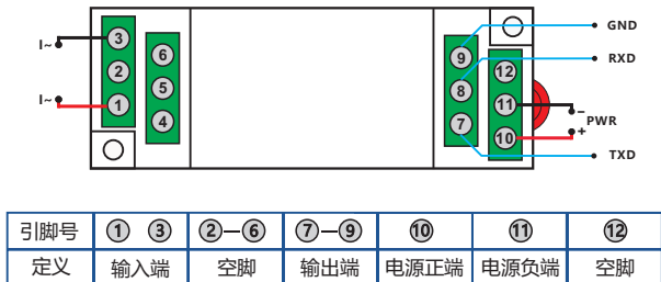
RS-232接线图:
