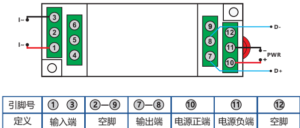
RS-485接线图:
