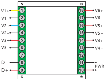
RS-485接线图：
