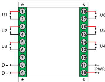
RS-485接线图：
